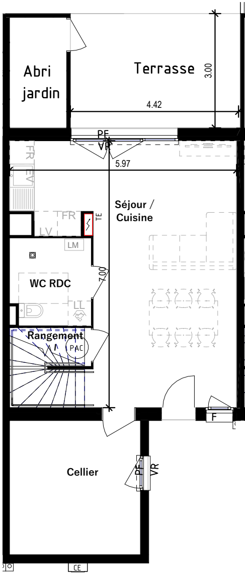
PLAN REZ-DE-CHAUSSEE - 6 ||| Ech: 1 : 100
