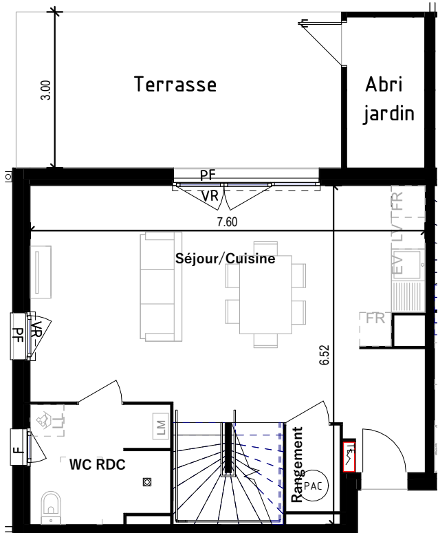
PLAN REZ-DE-CHAUSSEE - 2 ||| Ech: 1 : 100
