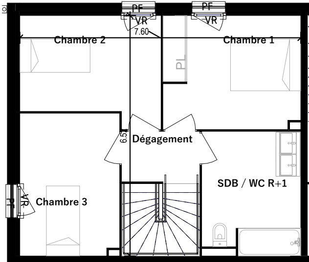
PLAN ETAGE - 2 ||| Ech: 1 : 100
